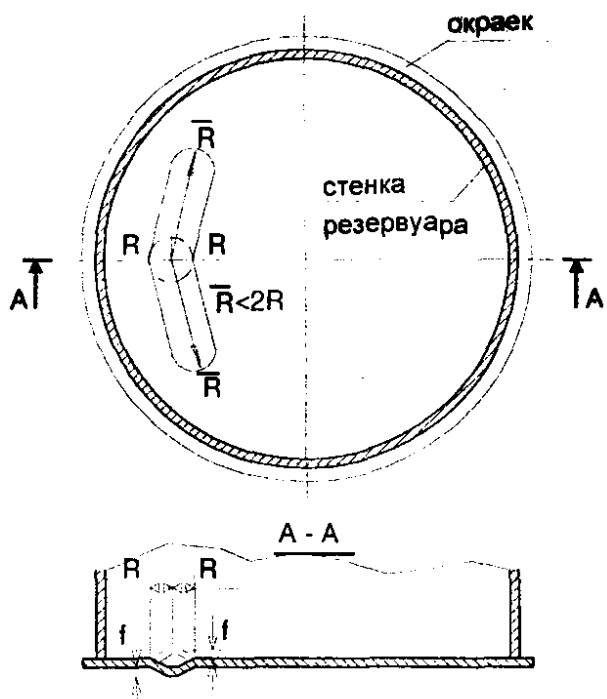
Р - ширина просадки f - глубина просадки Фиг. 5-3. Просадка края
